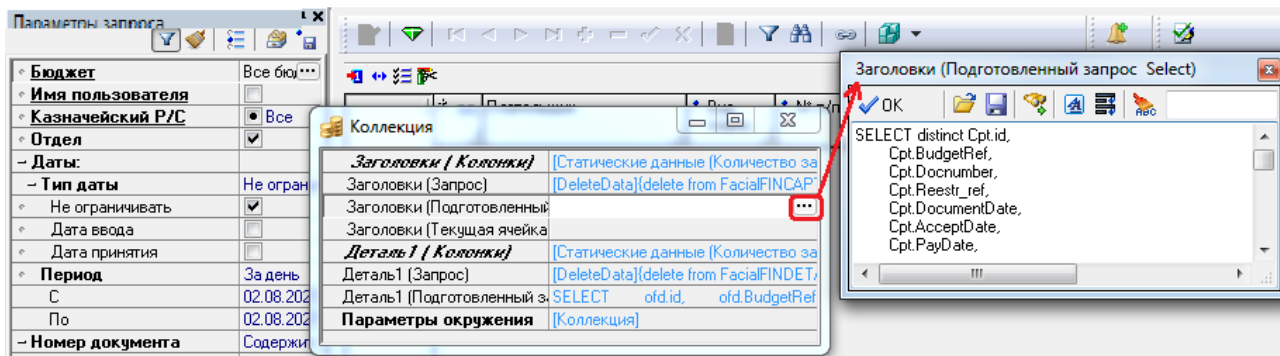
Рис. 3.51. Вид вызываемого окна «Коллекция» с перечнем полей и соответствующей модальной формой
