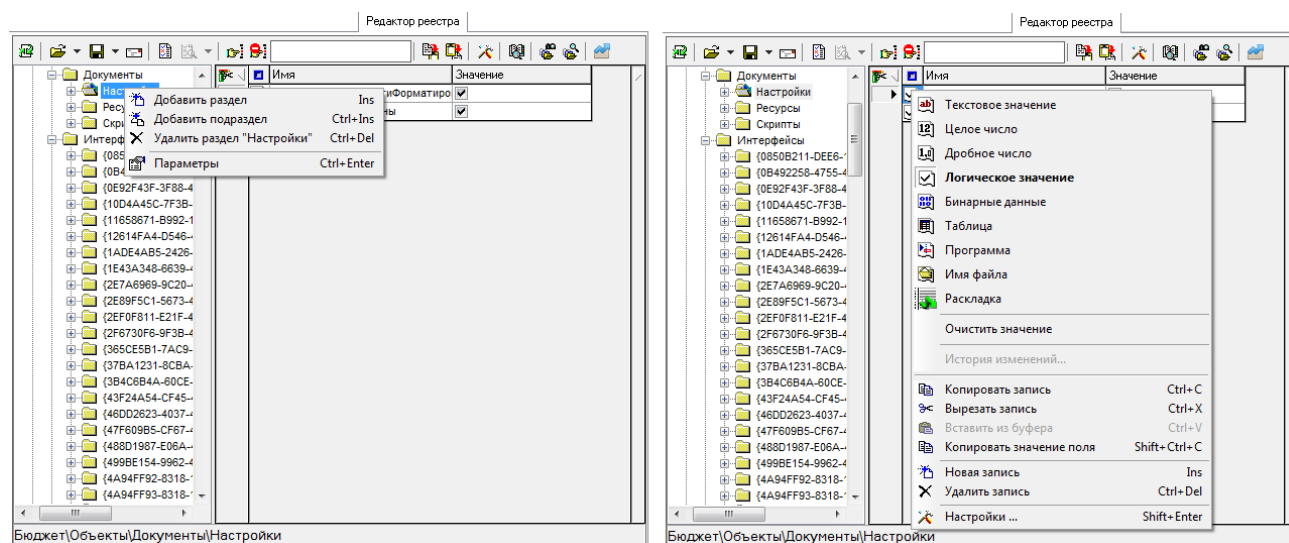
Рис. 3.31. Дерево реестра и контекстное меню дерева реестра (слева), таблица параметров и контекстное меню таблицы параметров (справа)
