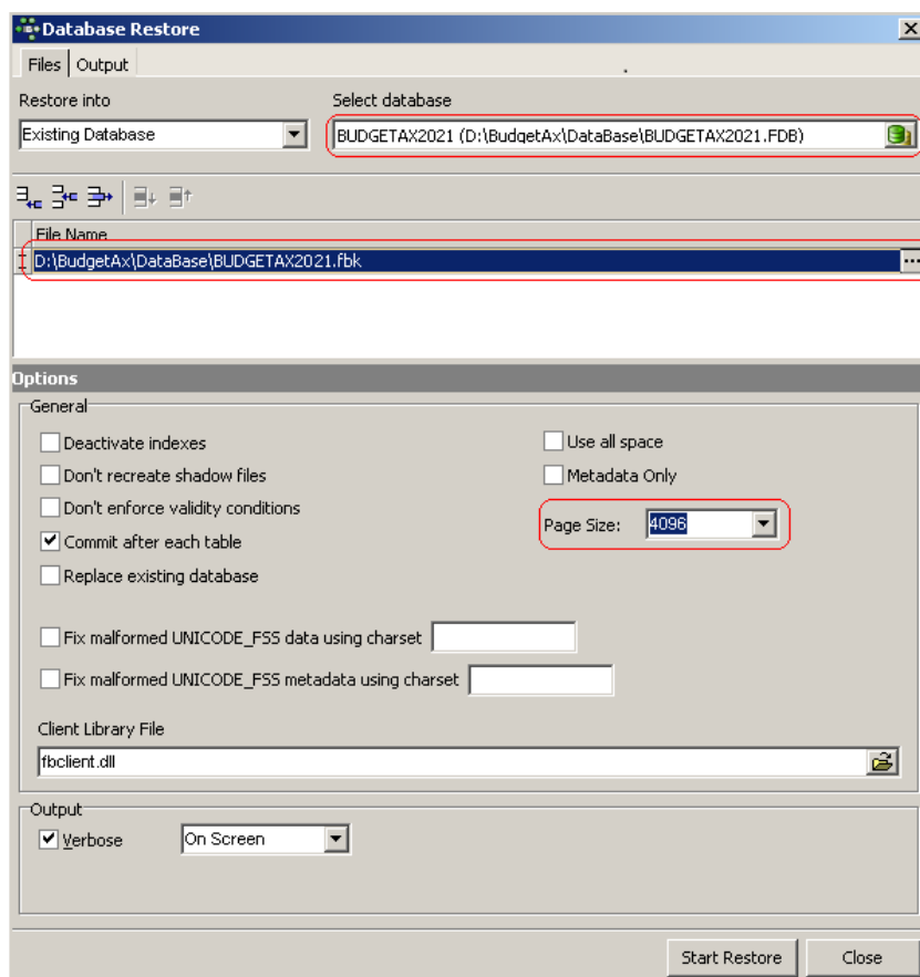
Рис. 2.3. Вид окна «Database Restore» («Восстановление БД»)
