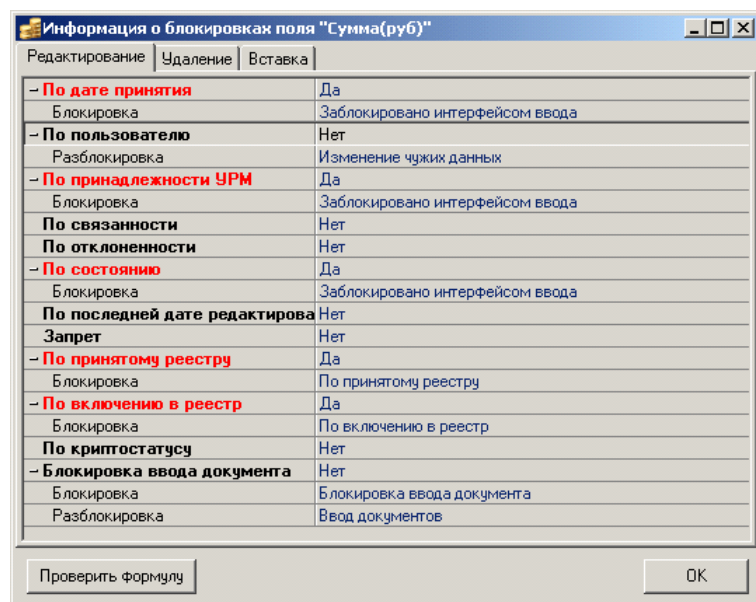
Рис. 1.56. Пример информационного окна для поля «Сумма(руб)» интерфейса (03.02) «Выбытия по п\п» РМ «Казначейство»
