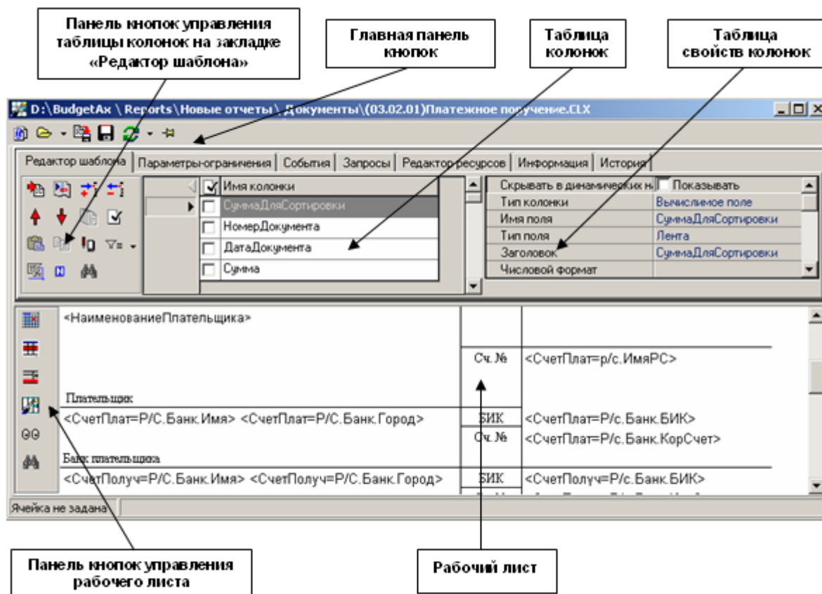
Рис. 4.17. Окно редактора печатного вида документа CellsEdit.exe на закладке «Редактор шаблона»
