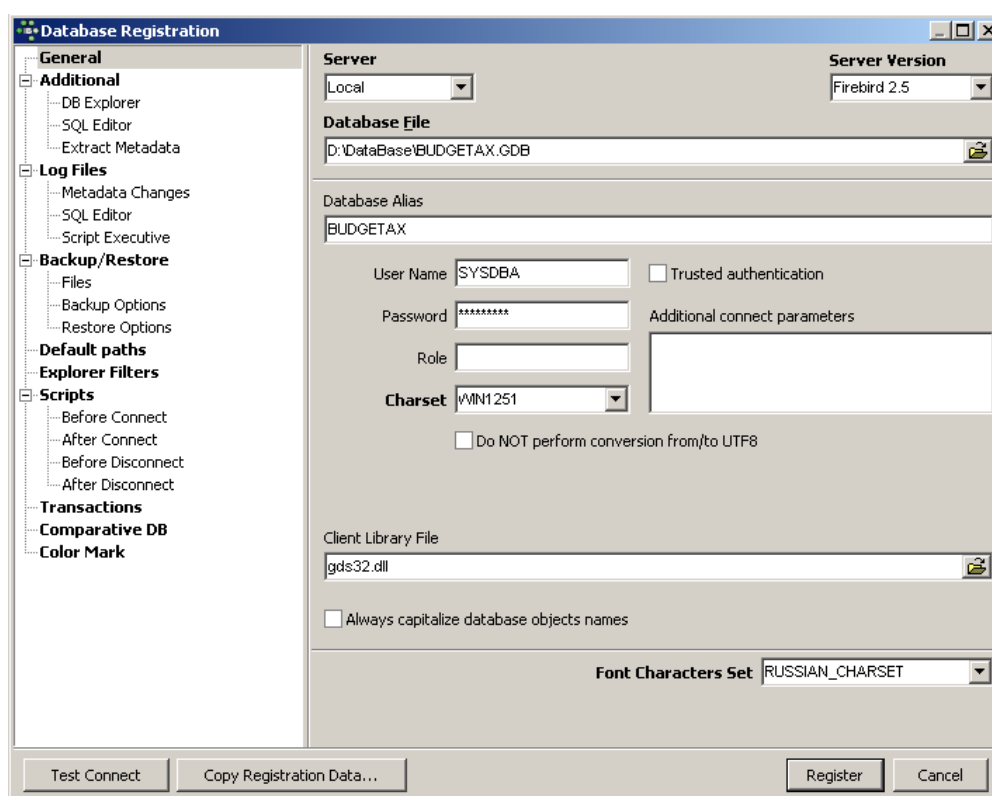
Рис. 1.39. Окно IBExpert для регистрации базы данных под управлением СУБД Firebird
