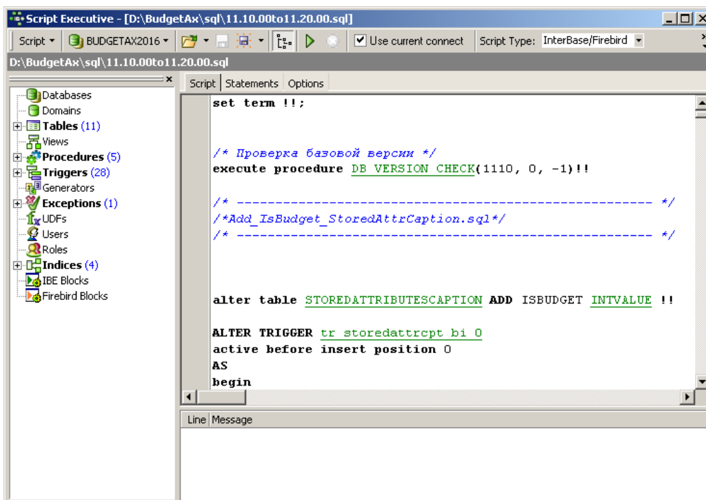
Рис. 2.4. Окно «Script Executive» утилиты IBEExpert
